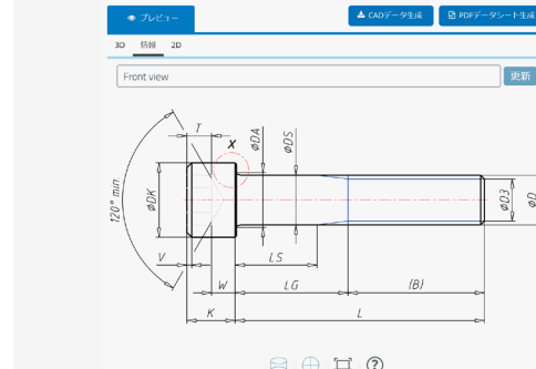
図4 平面図
