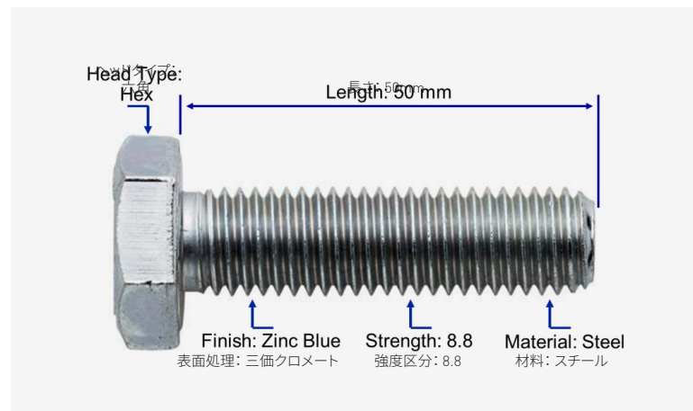
図1 六角ボルトDIN 933 M10x50mm 強度区分8.8 三価クロメート
