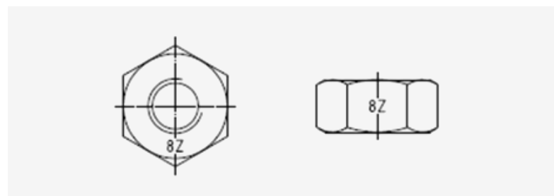
図11 コーティング後に公差位置6AZにオーバーサイズでタップされた溶融亜鉛メッキナットのマーキングの例
