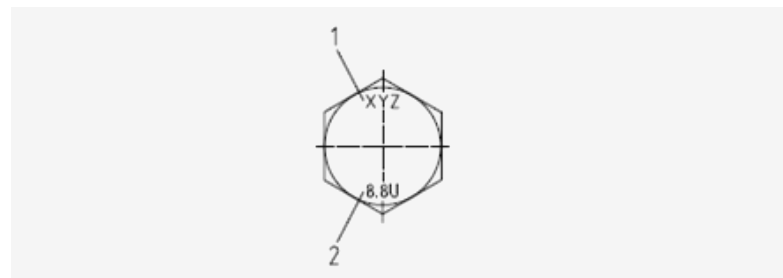
図10 コーティング前の溶融亜鉛メッキボルトおよびねじの公差クラス6az未満のねじのマーキングの例
